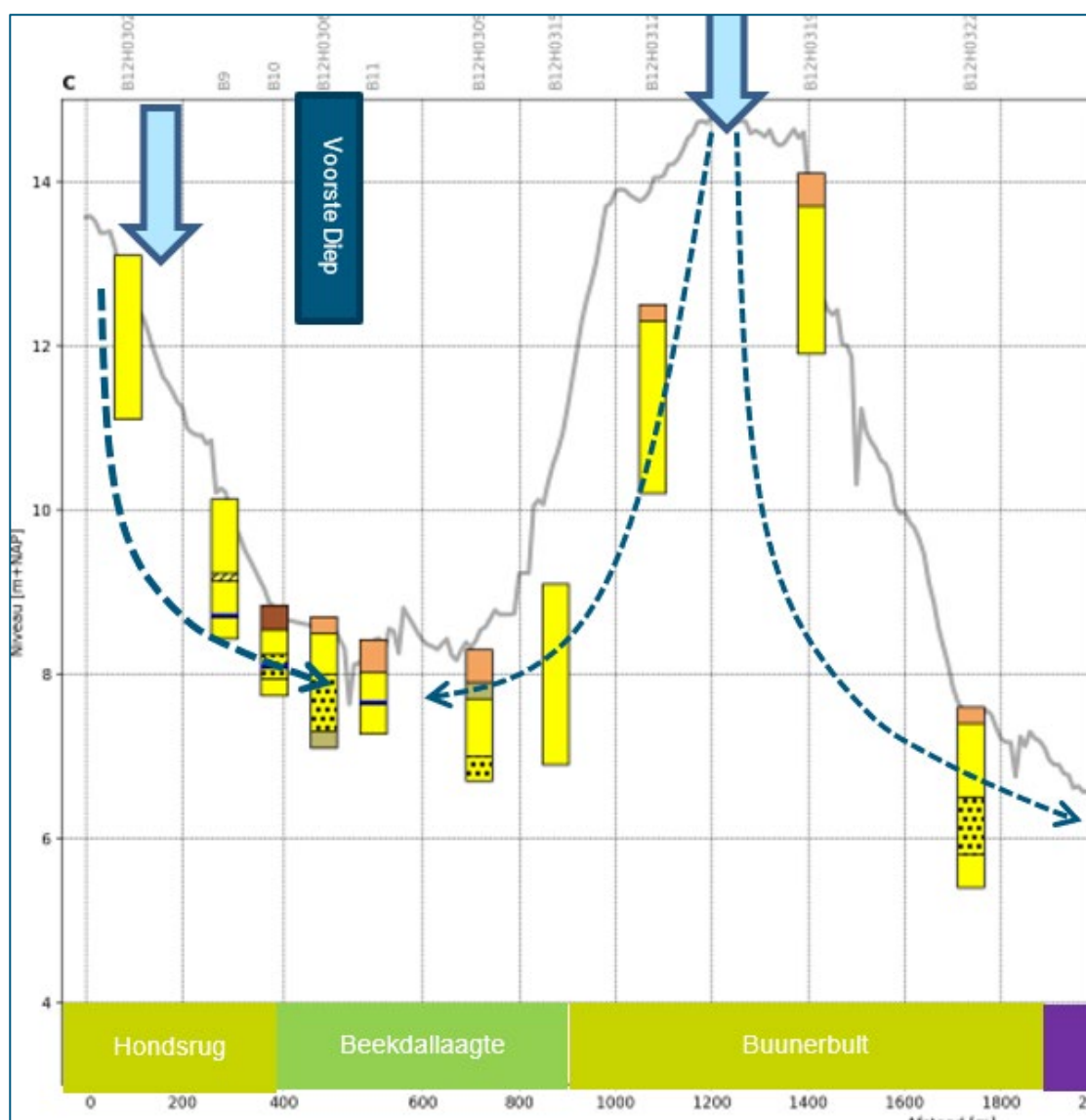
Figuur 4-5 Schematische weergave grondwaterstroming Bronnegemaden.
