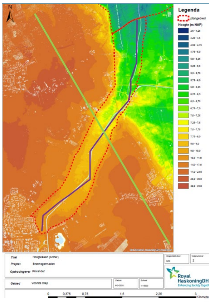
Figuur 3-1 Hoogtekaart Bronnegermaden met in paars het lengteprofiel en groen een dwarsdoorsnede (zie Figuur 3-2).
